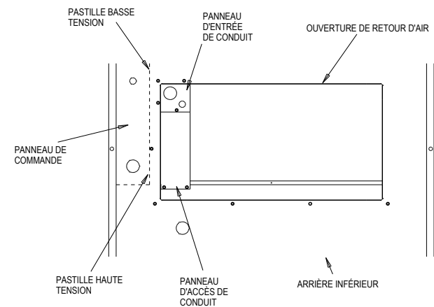
FIGURE 10 Installation du conduit flexible
