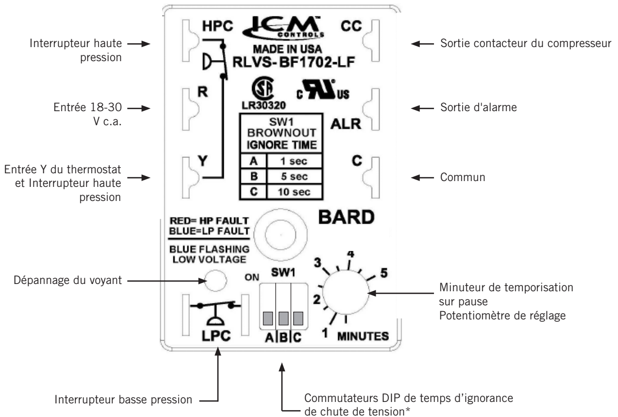
FIGURE 17 MODULE DE COMMANDE DU COMPRESSEUR
