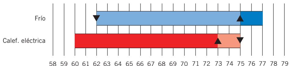
FIGURA 68 Control de la deshumidificación (°F)
