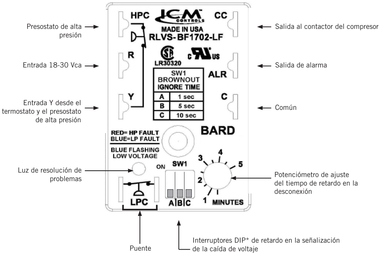
FIGURA 43 Módulo de control del compresor
