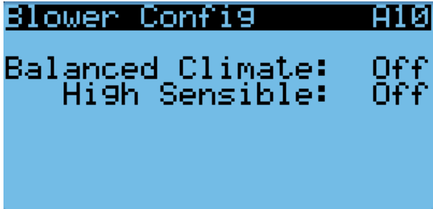
FIGURE 37 Activación/desactivación de la operación de alta sensato o operación Balanced Climate
