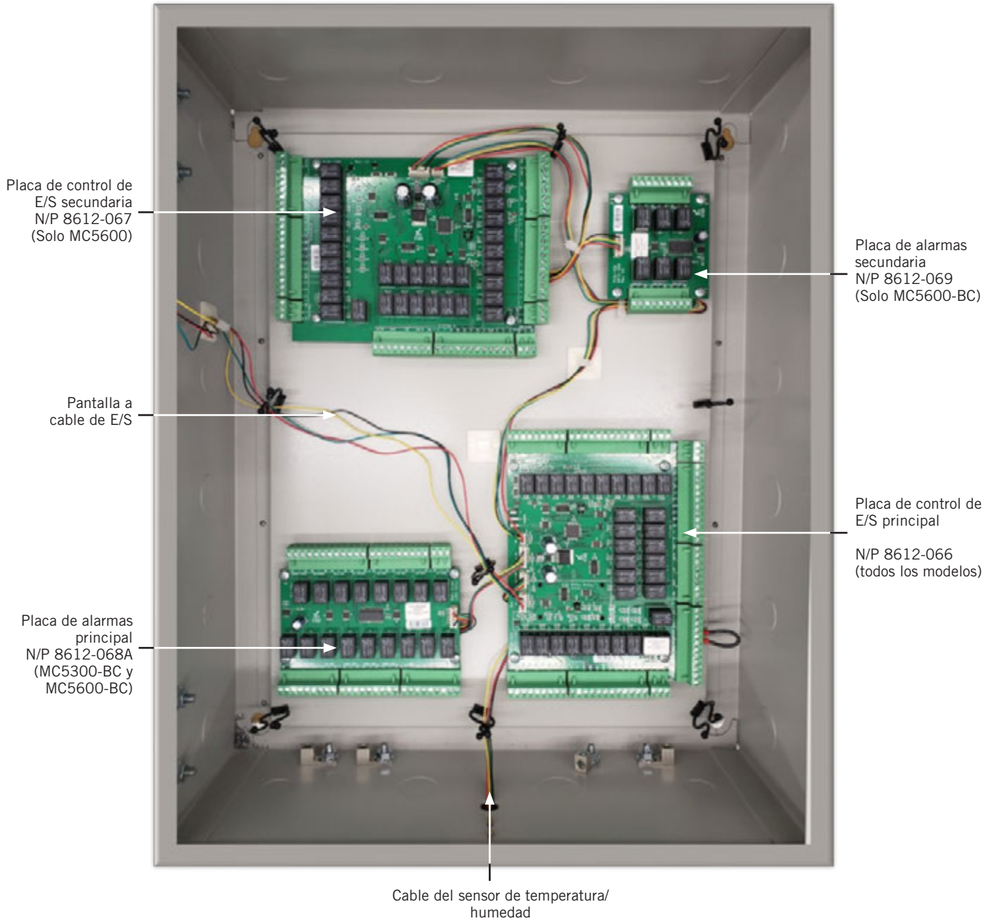
FIGURA 1 Ubicación habitual de los componentes de los controladores serie MC5000
