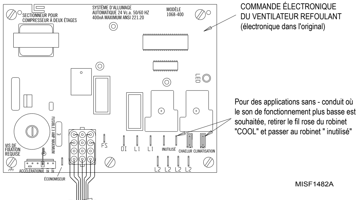
FIGURE 17 CARTE DE COMMANDE DE LA CHAUDIÈRE ET COMMANDE DU VENTILATEUR REFOULANT
