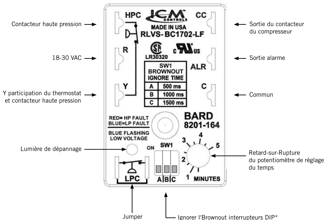
FIGURE 14 8201-164 MODULE DE COMMANDE DU COMPRESSEUR
