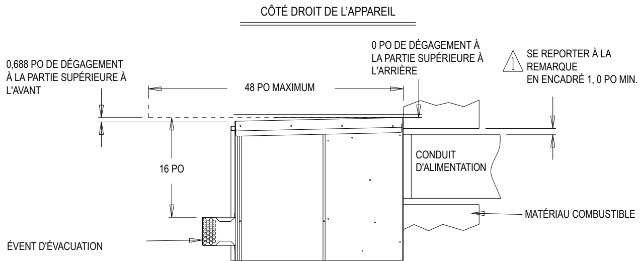
FIGURE 3 DÉGAGEMENTS PAR RAPPORT AUX MATÉRIAUX COMBUSTIBLES
