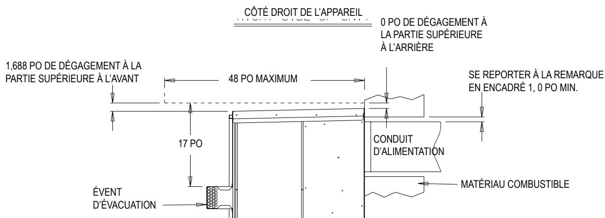
FIGURE 3 DÉGAGEMENTS PAR RAPPORT AUX MATÉRIAUX COMBUSTIBLES POUR LES MODÈLES W24G, W30G ET W36G
