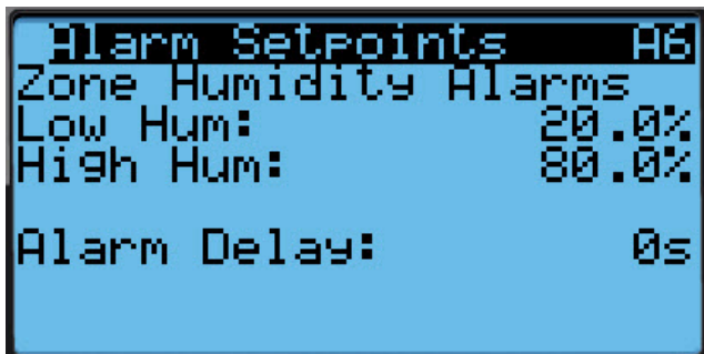
FIGURE 2.6 Réglage des points d'alarme d'humidité
