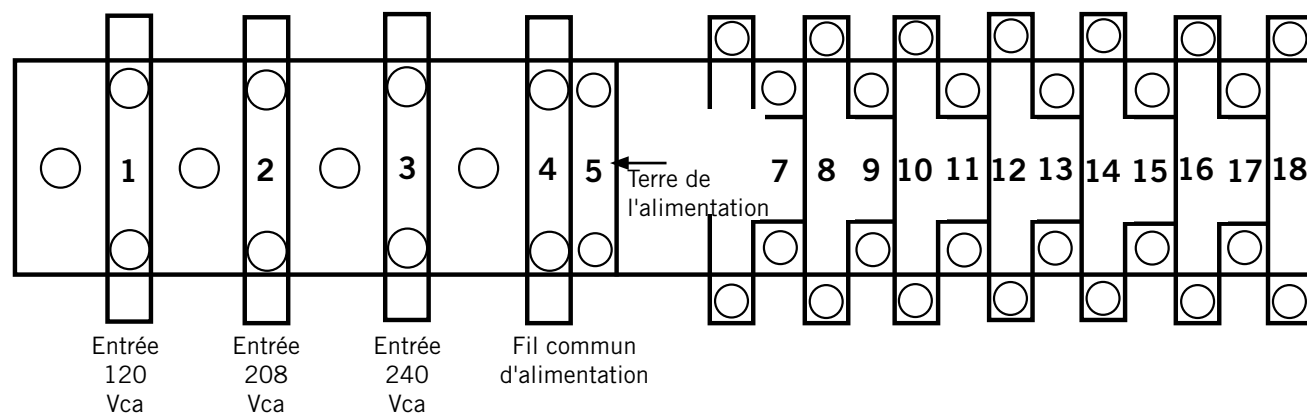
FIGURE 1.12 Installation du circuit du contrôleur LC6000
