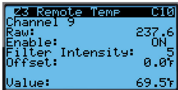
FIGURE 1.28 Activation/désactivation de la sonde distante de température zone 3
