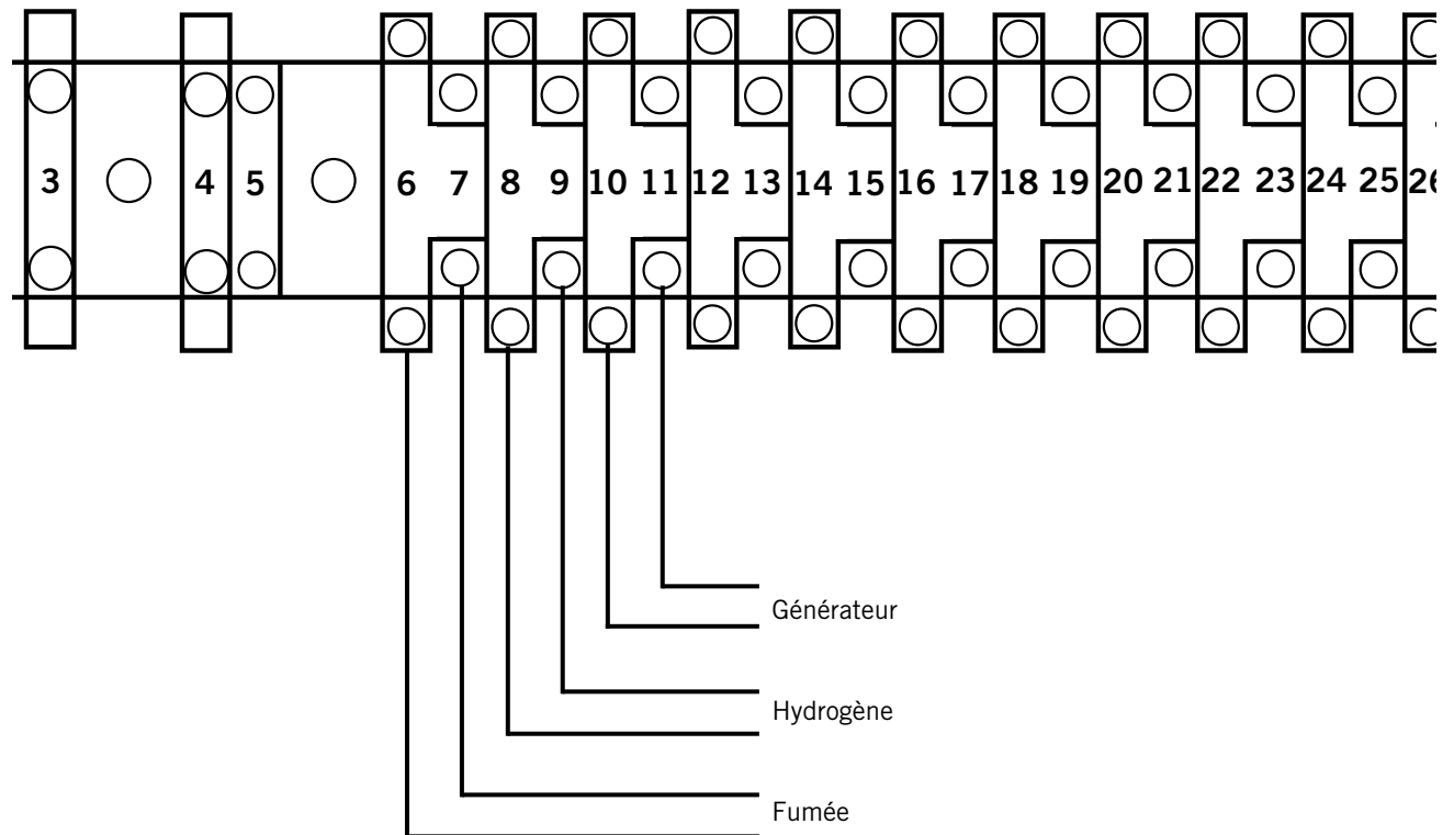
Connexions de la série LC6000-100 du détecteur de fumée, du détecteur d'hydrogène et de la mise en marche du générateur (le cas échéant)
