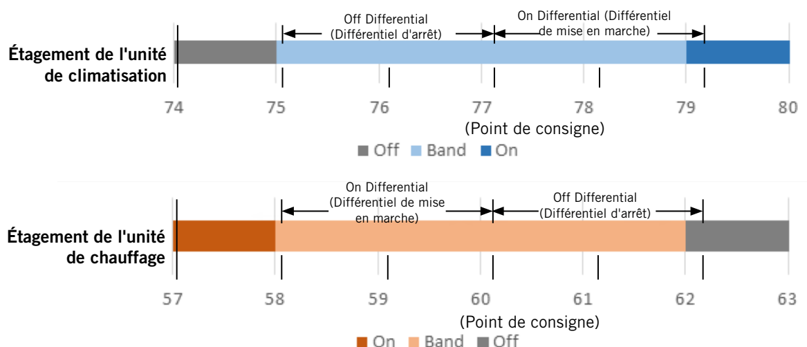
FIGURE 2.7 Étagement des unités par le LC6000
