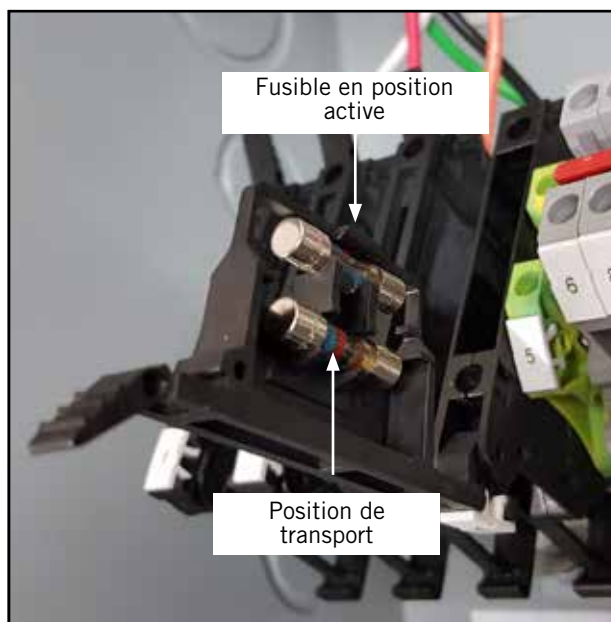
FIGURE 1.2 Bornes d'alimentation du LC6000 protégées par fusible
