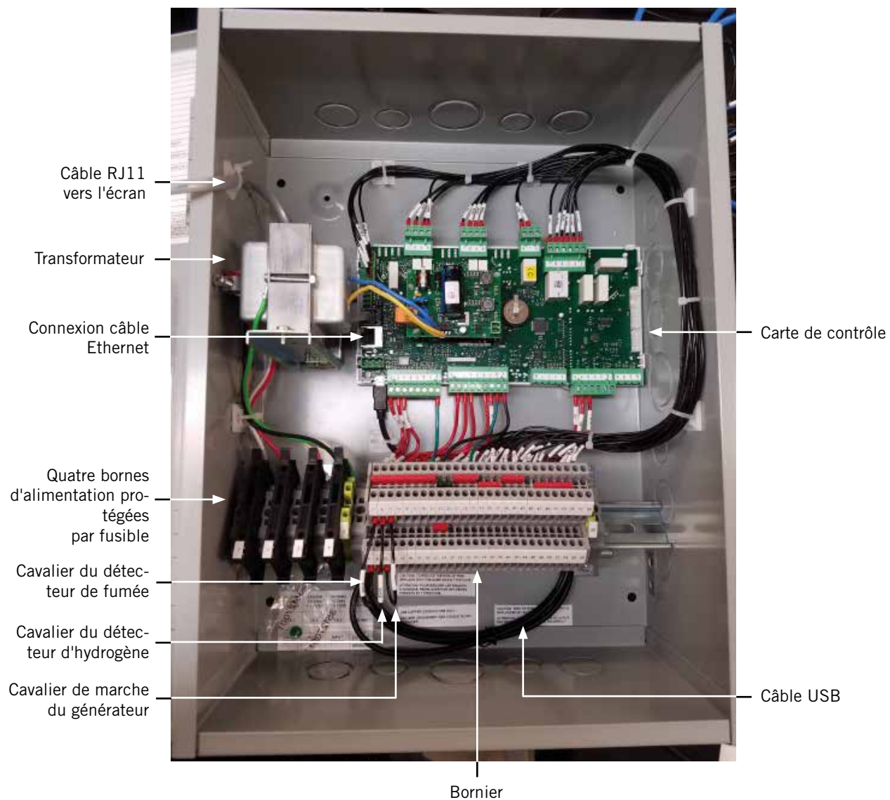
FIGURE 1.1 Emplacement des composants du LC6000
