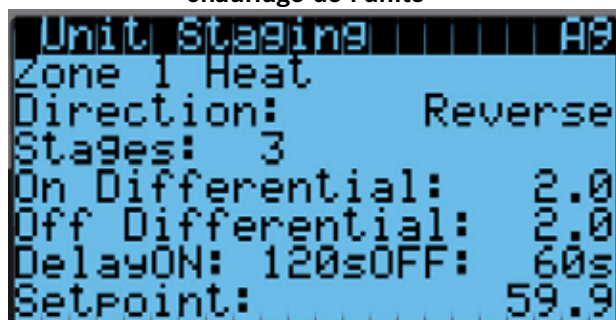
FIGURE 2.10 Modification des différentiels de chauffage de l'unité
