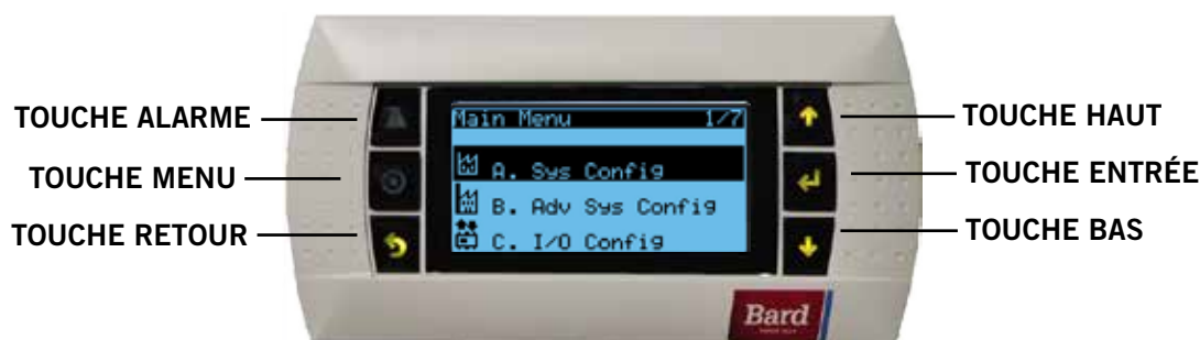
FIGURE 1.20 Écran et interface du contrôleur LC6000 (menu principal illustré)
