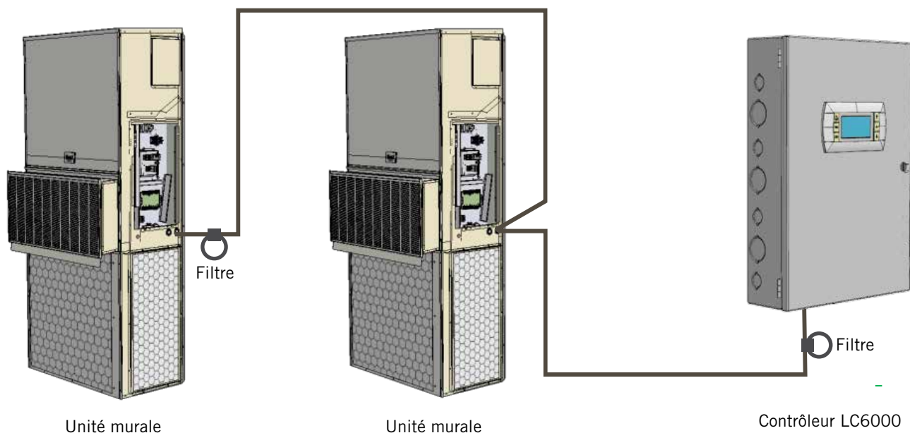
FIGURE 1.6 Câblage de communication (liaison série)
