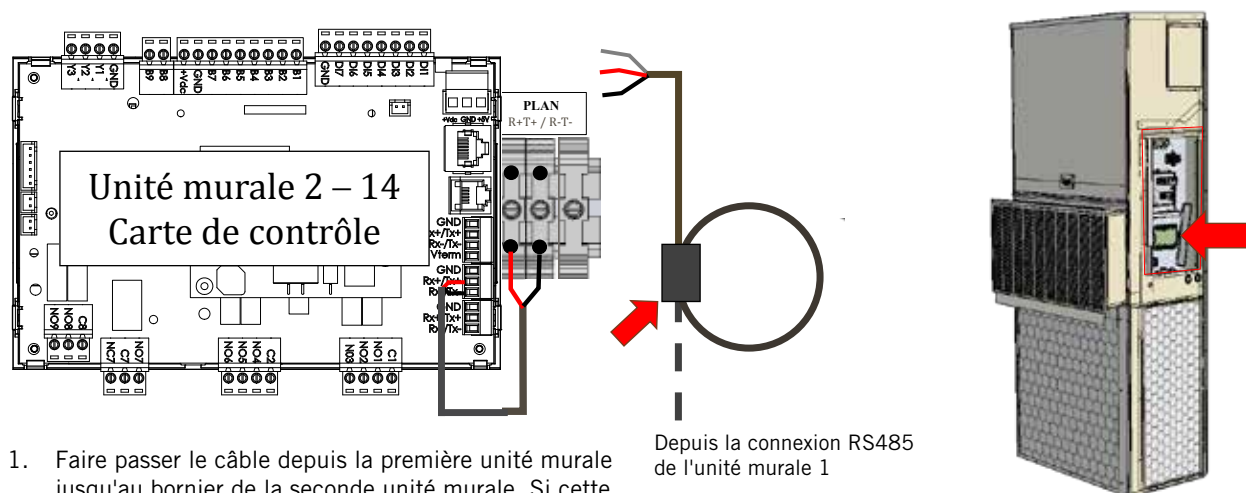
FIGURE 1.11 Câblage de communication : Terminaison au niveau des unités murales supplémentaires
