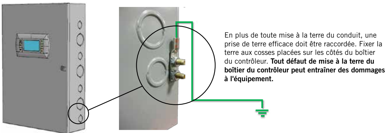
FIGURE 1.13 Points de masse du contrôleur
