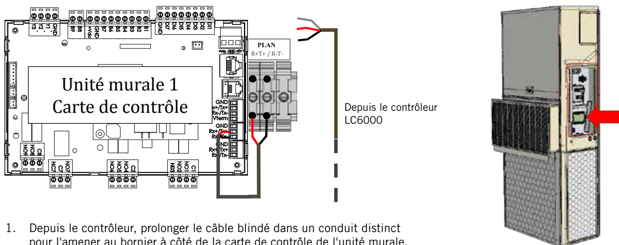
FIGURE 1.10 Câblage de communication : Terminaison au niveau de la première unité murale
