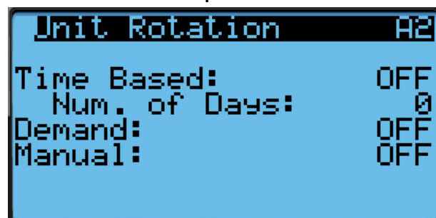
FIGURE 2.12 Modification des paramètres de rotation
