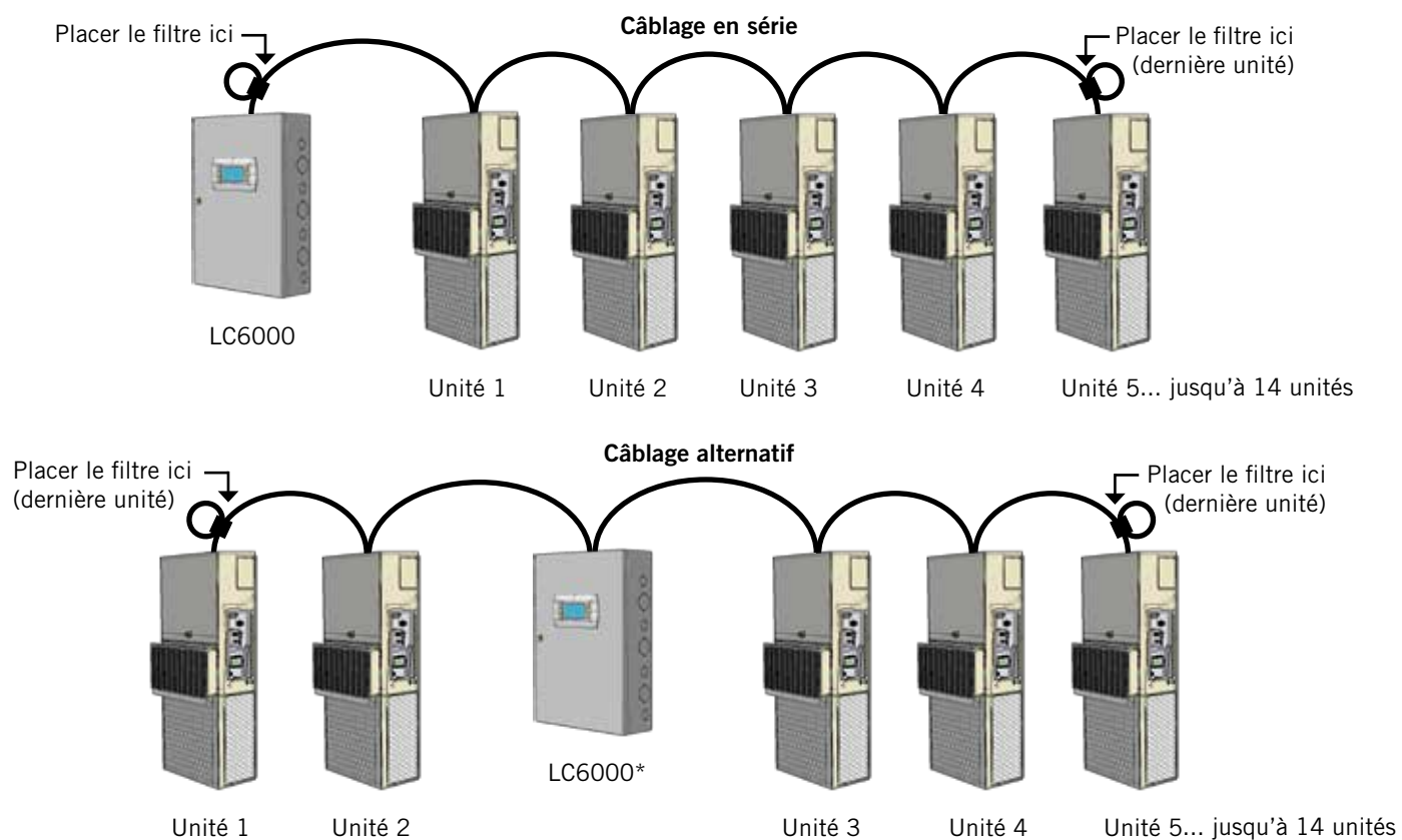
FIGURE 1.8 Positionnement des filtres de fil de communication (liaison en série ou alternative)
