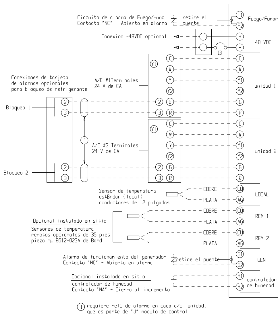
FIGURA 1 CONEXIONES DEL CONTROLADOR ETAPA 1 DE AIRES ACONDICIONADOS (SERIES WA/WL, W**A/W**L) - SIN ECONOMIZADOR
